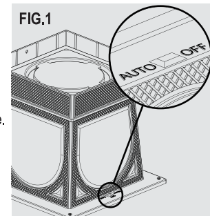
Instalación de postes de 6"x6"
