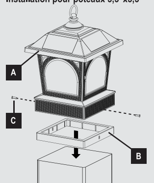
Installation pour poteaux 5,5"x5,5"
