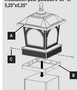
Installation pour poteaux 5"x5" et 5,25"x5,25"
